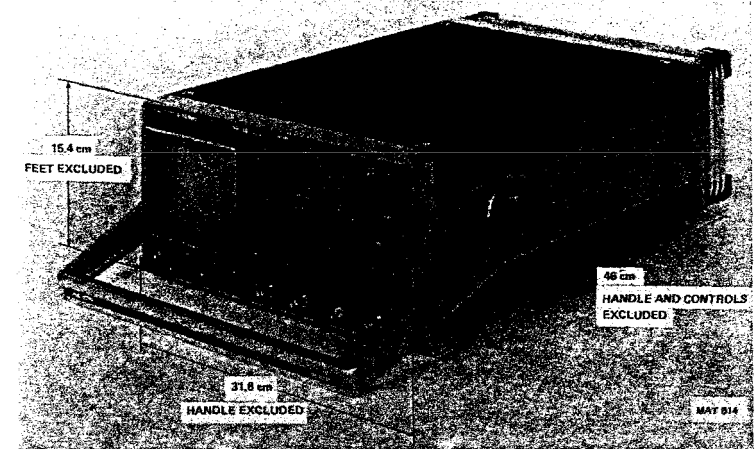
Fig. 4.2 Dimensions
